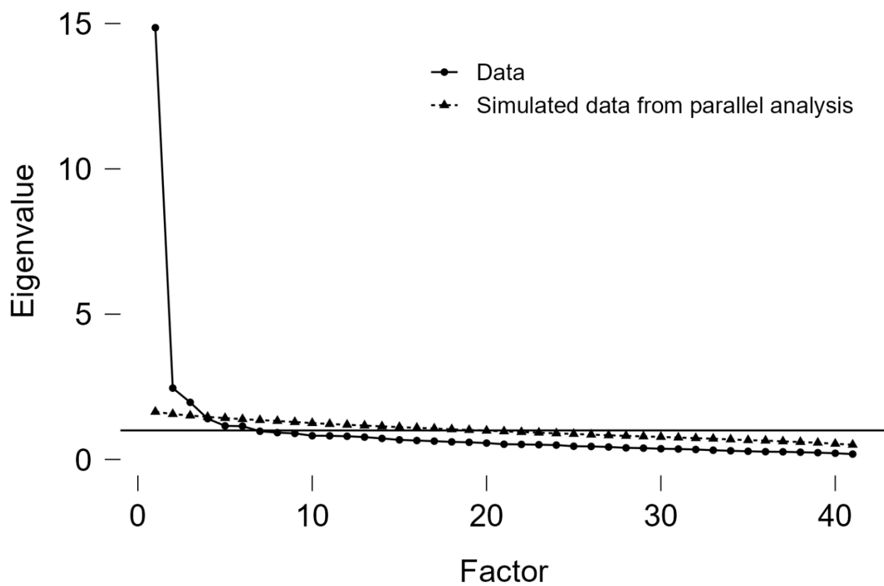
Grafikon 1. Rezultati scree testa i paralelne analize za Upitnik mitovi o nasilju
